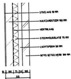
OPBOUW SPOUWMUUR MET ANDERE SAMENGEVEN
